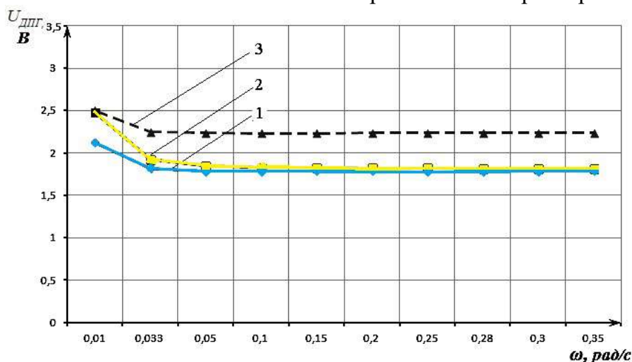
Рис. 9. Залежність амплітуди вихідної напруги ІП від частоти коливань вібростенда при різних напругах збудження: 1 - U_{IP} = \psi(\omega) при U_{ген} = 5 В; 2 - U_{IP} = \psi(\omega) при U_{ген} = 7 В; 3 - U_{IP} = \psi(\omega) при U_{ген} = 8 В
