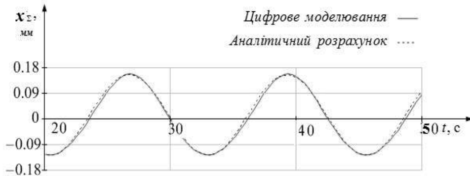
Рис. 5. Порівняння отриманих результатів вихідного сигналу (зміщення ІМ) при поступальних збуреннях із частотою \omega = \omega_0 цифрового моделювання із результатами аналітичних розрахунків
