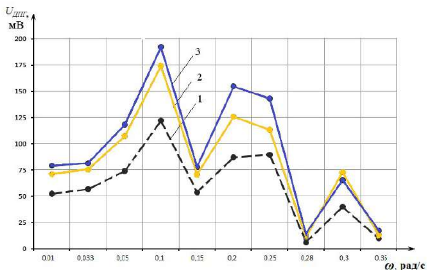
Рис. 8. Залежність вихідної напруги ДПГ від частоти коливань вібростенда при різних напругах збудження: 1 - U_{DPII} = \psi(\omega) при U_{ген} = 5 В; 2 - U_{DPII} = \psi(\omega) при U_{ген} = 7 В; 3 - U_{DPII} = \psi(\omega) при U_{ген} = 8 В
